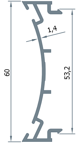
4238 ÇARPMA KAPI ADAPTÖR 0.470 kg/m.
