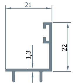
1990 "L" ÇİTA 0.206 kg/m.
