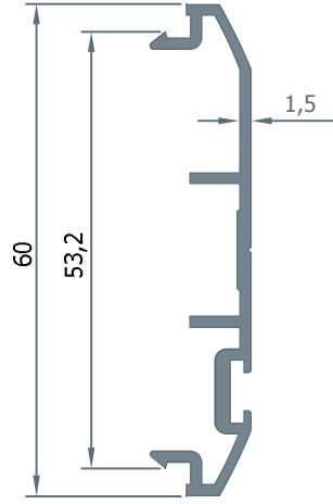
4237 ÇARPMA KAPI ADAPTÖR 0.440 kg/m.
