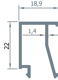
1985 CAM ÇİTASI 0.293 kg/m.
