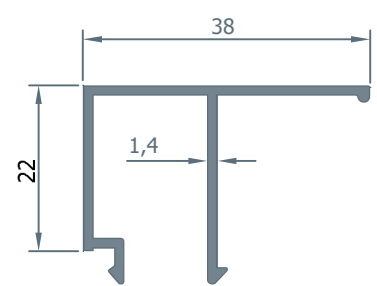
1992 CAM ÇİTASI 0.360 kg/m.
