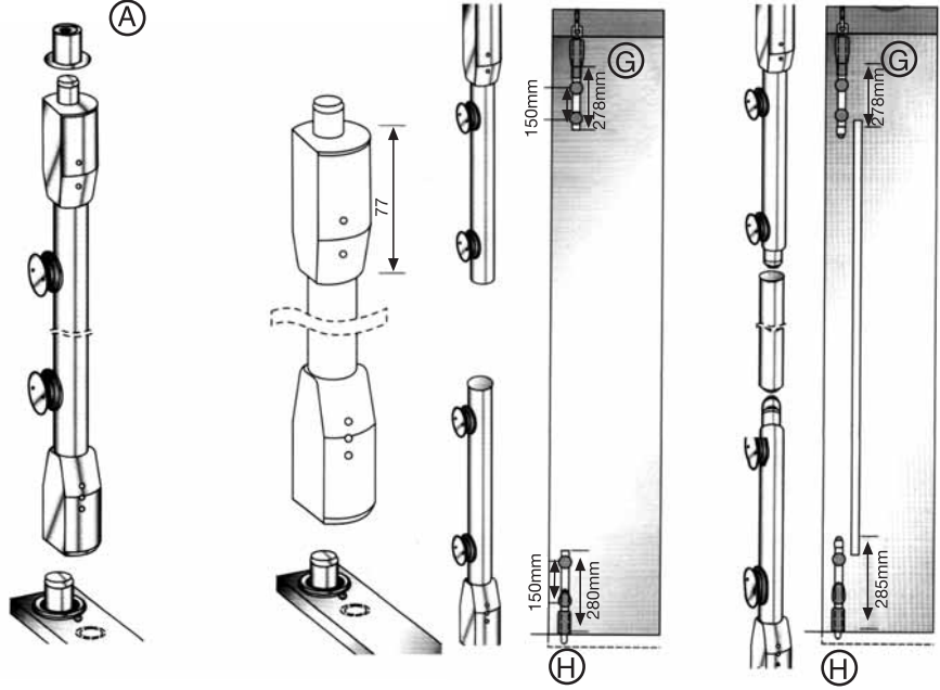
A- Tavan bağlantısı, G- Tavan pivot kasa bağlantısı, H- Zemin pivot bağlantısı,
