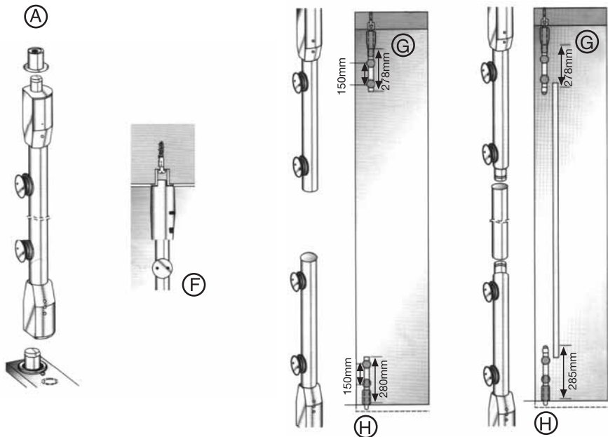
A- Tavan bağlantısı, G- Tavan pivot kasa bağlantısı, H- Zemin pivot bağlantısı, F- Tavan montajı
