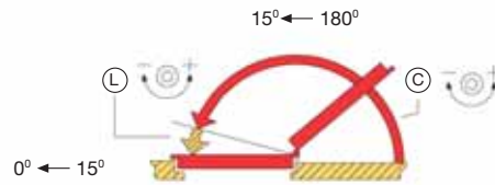
Kapanma ve Tokatlama Hız Ayarı Closing and Latching Speed
