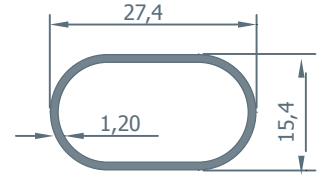
614 0.223 kg/m.
