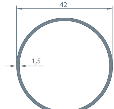
549 0.518 kg/m.
