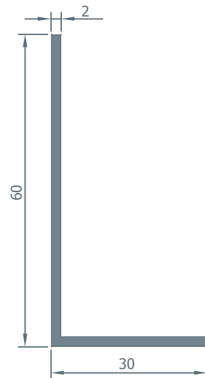
601.19 0.477 kg/m.
