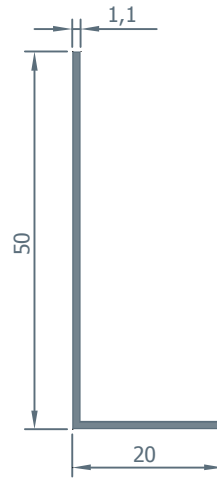
2165 0.206 kg/m.
