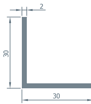
601.14 0.315 kg/m.
