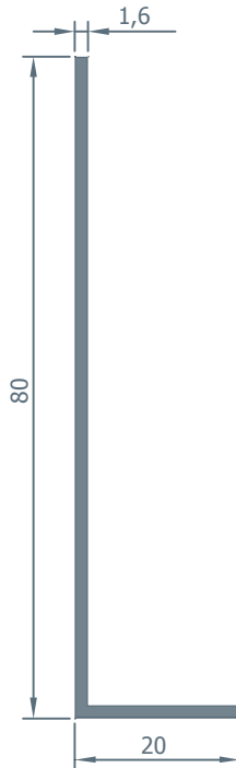
601.21 0.427 kg/m.
