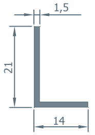
601.16 0.136 kg/m.
