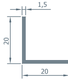
601.15 0.157 kg/m.
