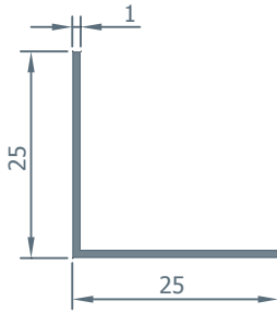
104 0.133 kg/m.
