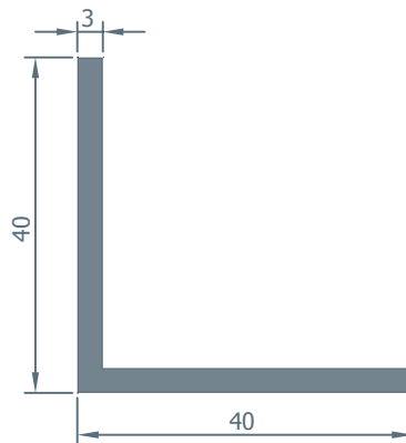
601.09 0.626 kg/m.
