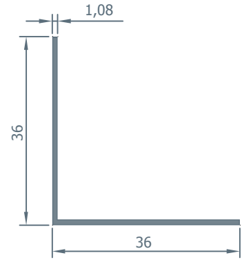
601.17 0.208 kg/m.
