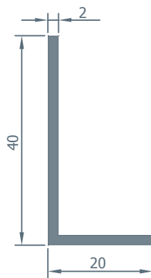
601.24 0.314 kg/m.
