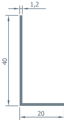
105 0.192 kg/m.
