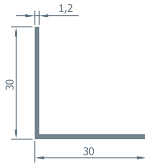
106 0.191 kg/m.
