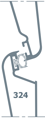
1.1 Detayı Details
