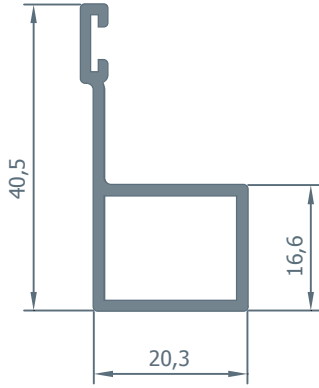
2052 0.350 kg/m.
