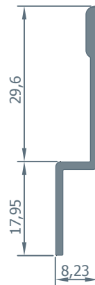
4461 0.271 kg/m.
