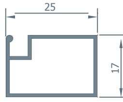
2051 0.247 kg/m.
