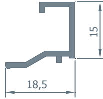
2092 0.179 kg/m.
