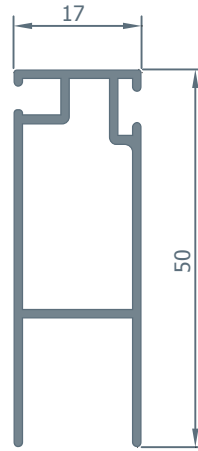
2313 0.499 kg/m.
