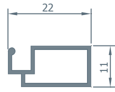
2910 0.195 kg/m.
