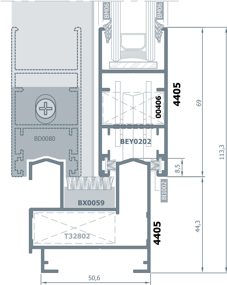
2.2 Detayı Details
