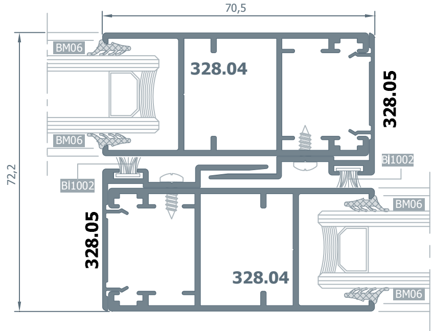
1.1 Detayı Details
