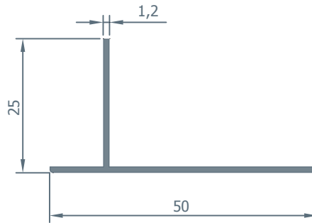
2824 0.240 kg/m.
