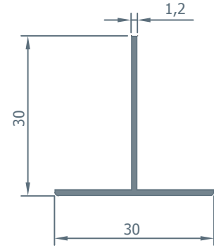
1387 0.191 kg/m.
