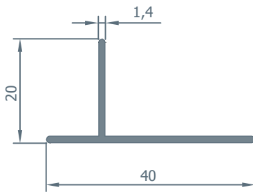
2753 0.221 kg/m.
