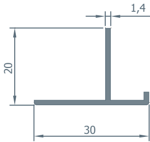
2682 0.192 kg/m.
