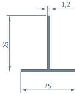
2820 0.159 kg/m.
