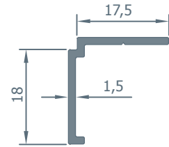
0008 0.161 kg/m.
