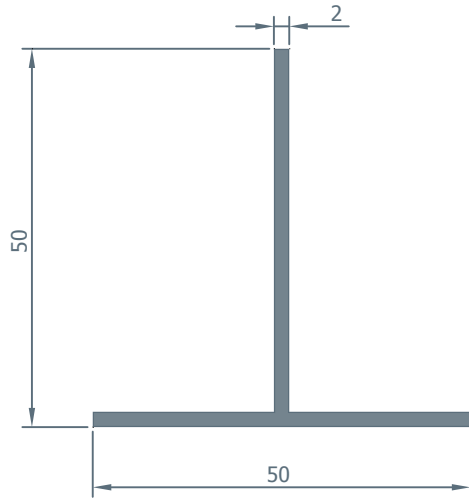
0035 0.530 kg/m.
