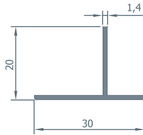
2732 0.185 kg/m.
