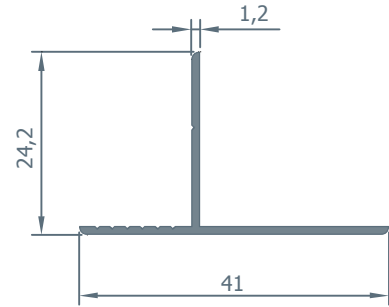
2685 0.206 kg/m.
