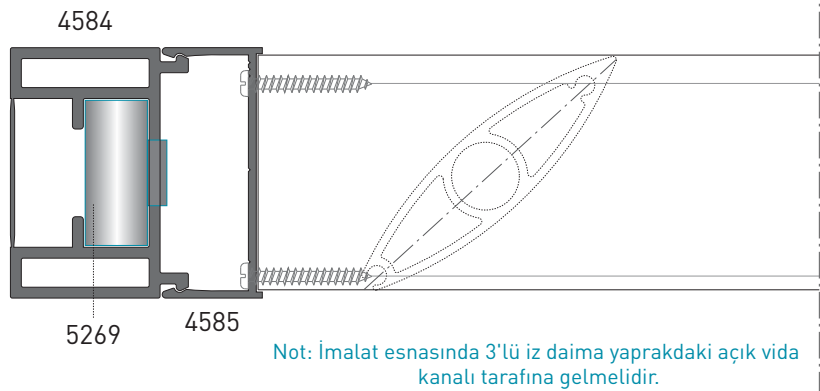
YATAY KESİT
