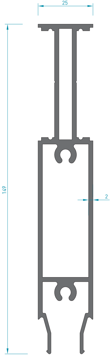
5493 KASA ARKA PROFİLİ ( 25'LİK) 2.250 kg/mt Jx : 153.31 cm 4 Jy : 5.73 cm 4
