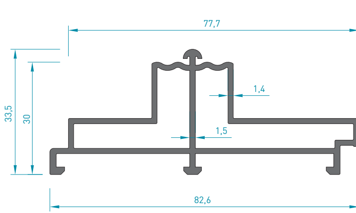
1956 SÜRME SİSTEM KASA 1.005 kg/mt Jx : 19.02 cm 4 Jy : 2.76 cm 4
