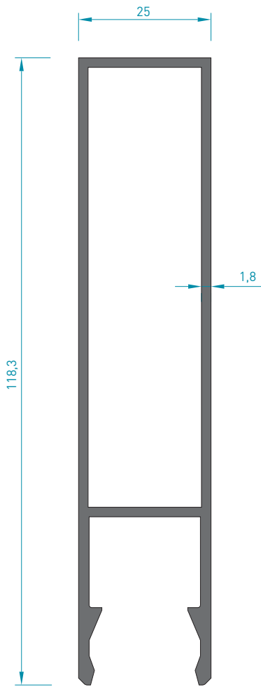
5495 KASA UÇ PROFİLİ ( 25'LİK) 1.455 kg/mt Jx : 72.83 cm 4 Jy : 6.40 cm 4
