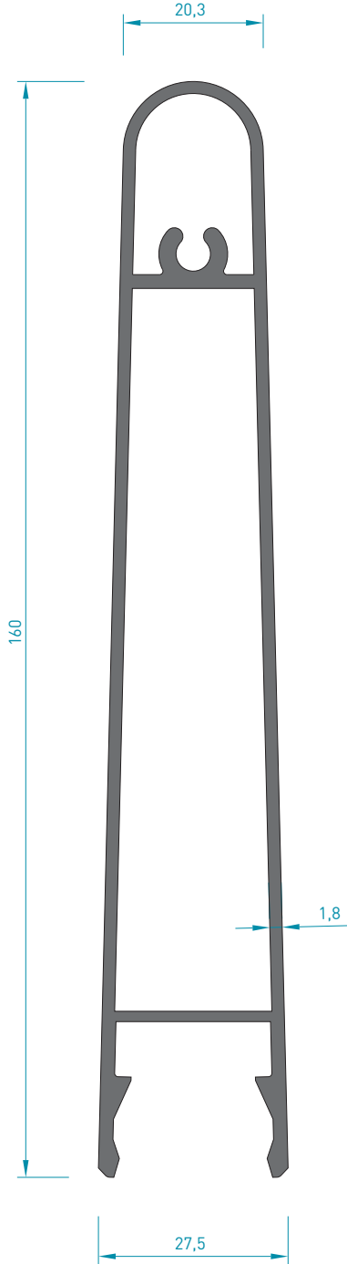
2683 GÜNEŞ KIRICI YAPRAK PROFİL 1.965 kg/mt Jx : 174.25 cm 4 Jy : 7.52 cm 4
