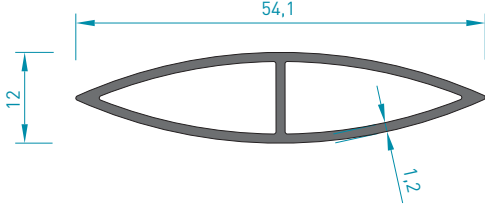
1952 YAPRAK PROFİL 0.380 kg/mt
