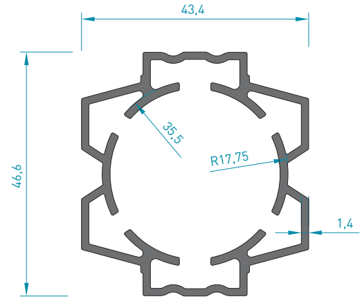
4723 ORTA BAĞLANTI 0.965 kg/mt
