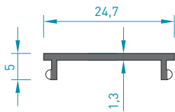
5489 ANKRAJ KAPAK 0.115 kg/mt
