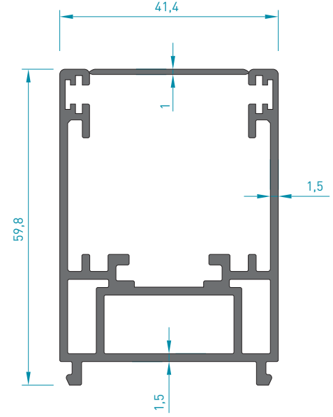
1961 SÜRME SİSTEM KANAT 1.240 kg/mt Jx : 16,10 cm 4 Jy : 11.24 cm 4
