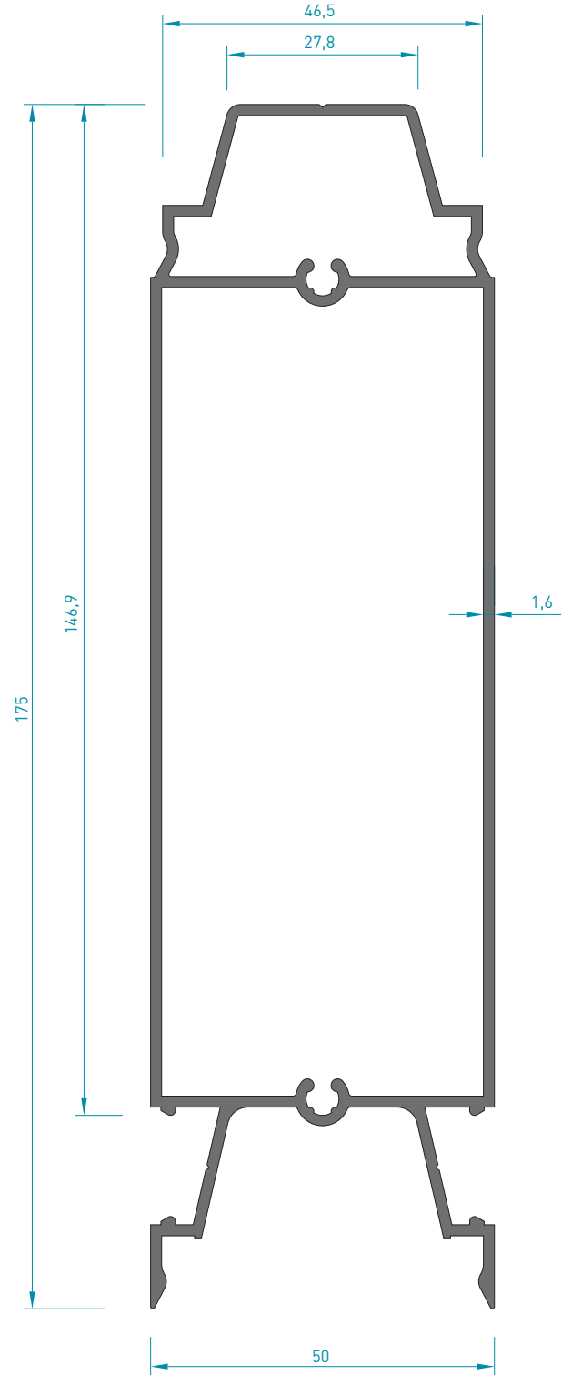
2491 ORTA BAĞLANTI 2.245 kg/mt Jx : 260.80 cm 4 Jy : 34.00 cm 4
