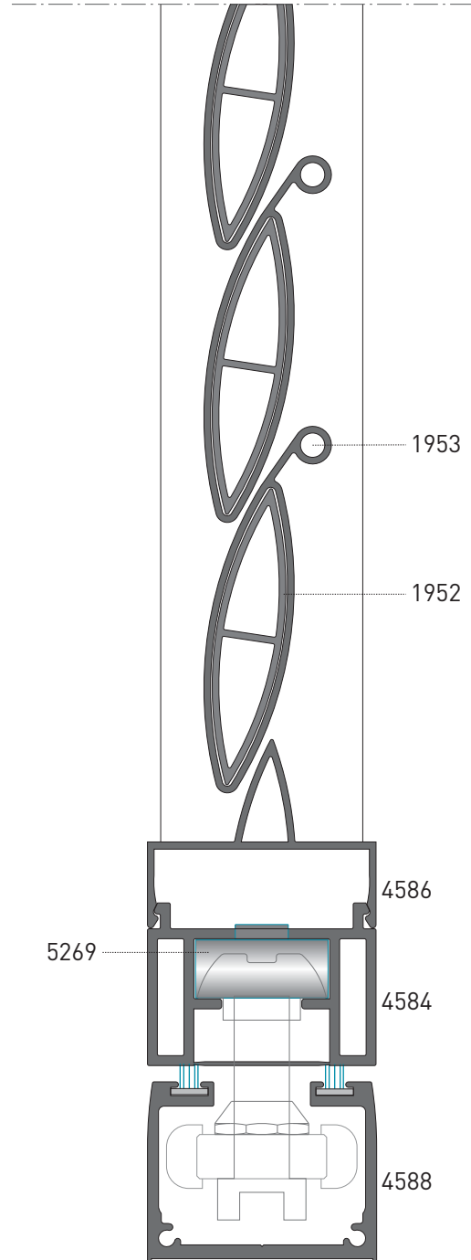
DÜŞEY KESİT (ALT DETAY)
