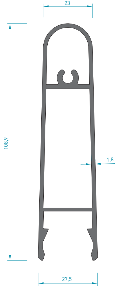
5499 GÜNEŞ KIRICI YAPRAK PROFİL 1.500 kg/mt Jx : 58.61 cm 4 Jy : 5.85 cm 4
