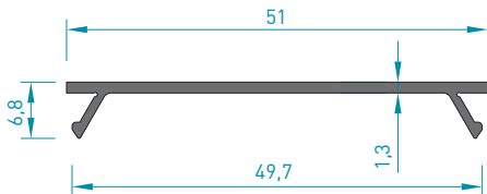
5488 KASA KAPAK PROFİLİ 0.220 kg/mt
