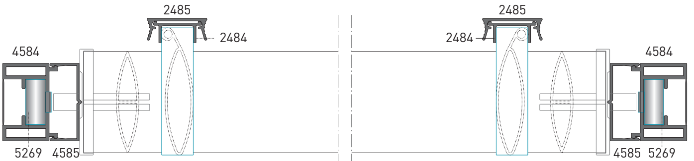
YATAY KESİT
