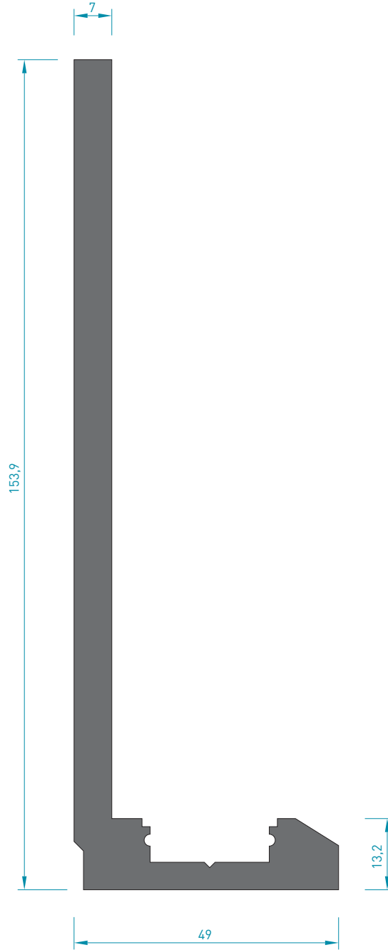
5490 " L " ANKRAJ 3.820 kg/mt Jx : 351.85 cm 4 Jy : 16.24 cm 4
