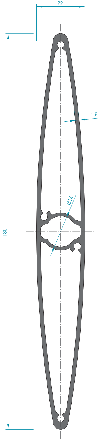
5433 GÜNEŞ KIRICI PROFİLİ 2.055 kg/mt Jx : 195.21 cm 4 Jy : 4.23 cm 4
