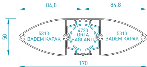
MONTAJ YAPILMIŞ DURUMDA 1 MT +/- 2.955 kg/mt
