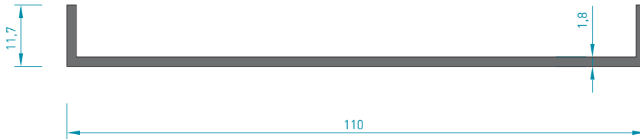
5435 GÜNEŞ KIRICI KASA 0.635 kg/mt Jx : 30.40 cm 4 Jy : 0.14 cm 4
