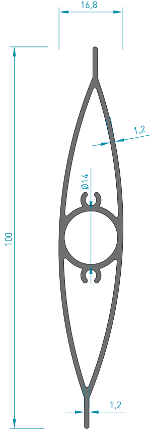
5436 GÜNEŞ KIRICI PROFİLİ 0.805 kg/mt Jx : 16.45 cm 4 Jy : 0.80 cm 4
