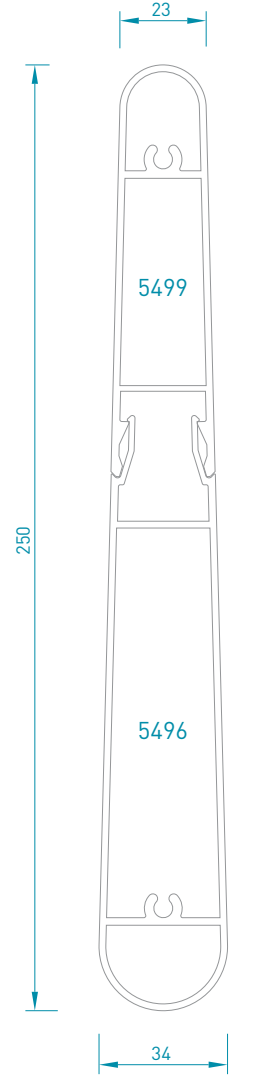
MONTAJ DETAYI ÖLÇEK: 1/2
