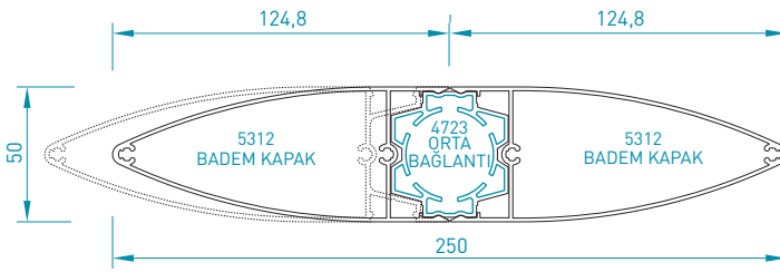
MONTAJ YAPILMIŞ DURUMDA 1 MT +/- 3.515 kg/mt
