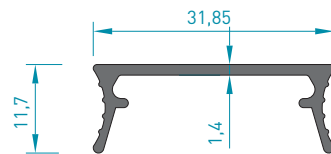
2485 TUTAMAK PROFİL 0.210 kg/mt
