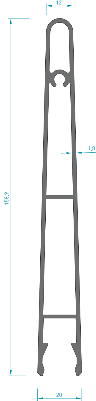
5498 GÜNEŞ KIRICI YAPRAK PROFİL 1.880 kg/mt Jx : 3.13 cm 4 Jy : 156.41 cm 4
