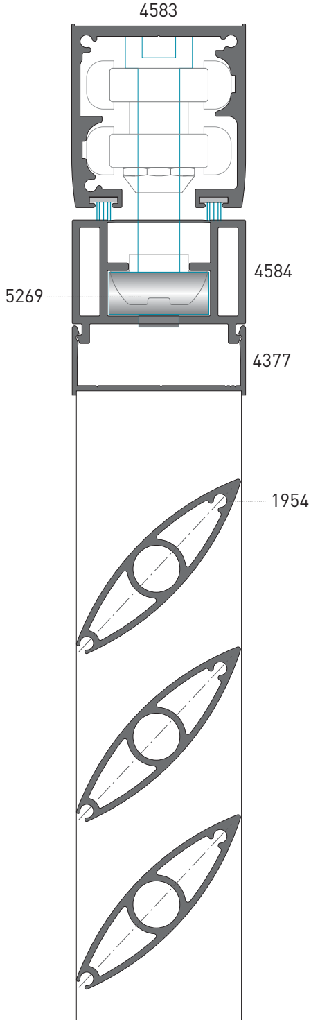
DÜŞEY KESİT
