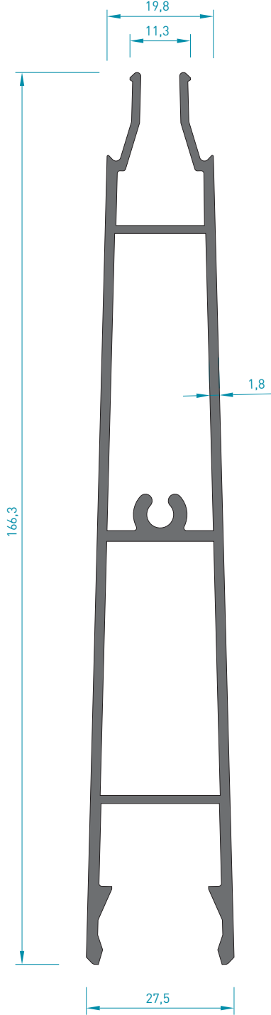
5497 GÜNEŞ KIRICI YAPRAK PROFİL 2.090 kg/mt Jx : 170.30 cm 4 Jy : 7.53 cm 4
