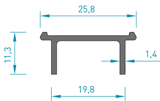
2484 TUTAMAK ALT PROFİL 0.170 kg/mt
