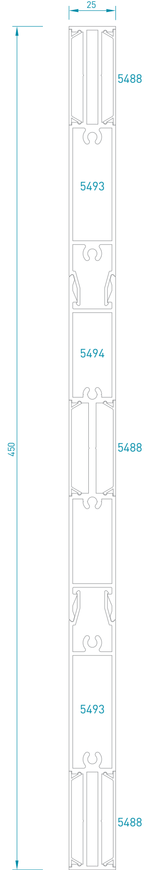
İNCE KASA MONTAJ DETAYI ÖLÇEK: 1/2
