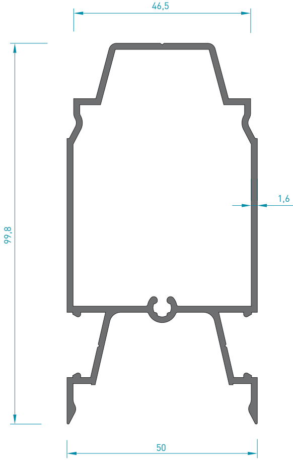
2490 ORTA BAĞLANTI 1.355 kg/mt Jx : 45.74 cm 4 Jy : 18.63 cm 4
