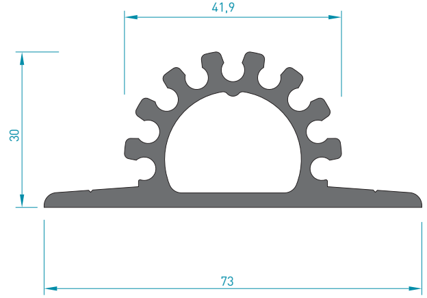
4888 GÜNEŞ KIRICI ALT BAĞLANTI APARATI 1.415 kg/mt Jx : 14.71 cm 4 Jy : 4.80 cm 4
