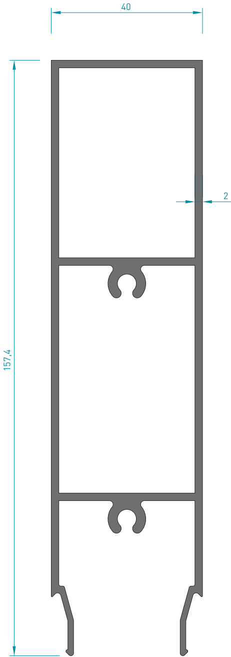
5491 KASA UÇ PROFİLİ ( 40'LIK) 2.550 kg/mt Jx : 24.21 cm 4 Jy : 191.98 cm 4
