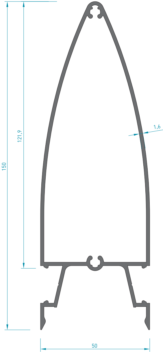
2492 ÜST KAPAK PROFİLİ 1.695 kg/mt Jx : 126.57 cm 4 Jy : 21.10 cm 4
