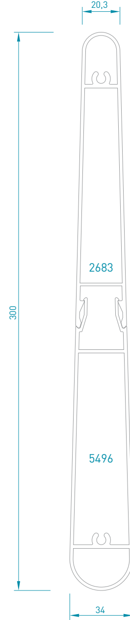
MONTAJ DETAYI ÖLÇEK: 1/2
