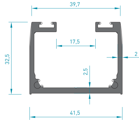
4588 ASKILI SİSTEM ALT RAY KASA 0.775 kg/mt Jx : 7.40 cm 4 Jy : 4.00 cm 4
