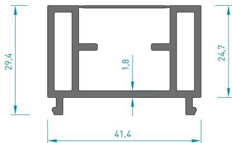
4584 ASKILI SİSTEM KANAT PROFİL 0.845 kg/mt Jx : 7.10 cm 4 Jy : 2.50 cm 4
