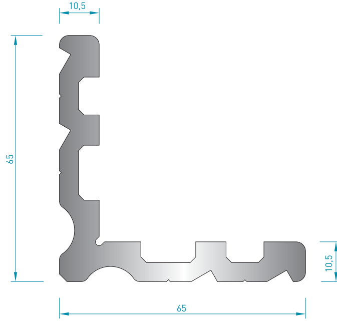
5269 KÖŞE TAKOZU 2.345 kg/mt
