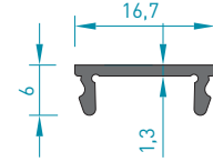
2839 YAN KAPAK PROFİLİ 0.095 kg/mt
