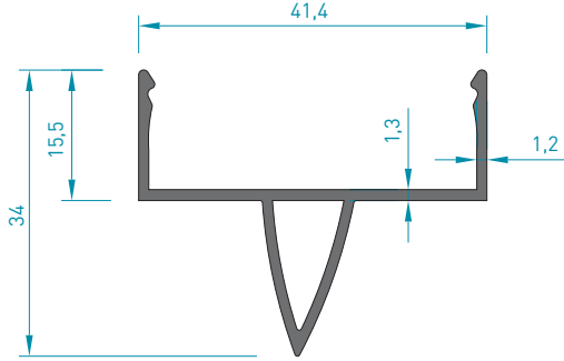
4586 ALT VE ÜST ÇITA 0.365 kg/mt
