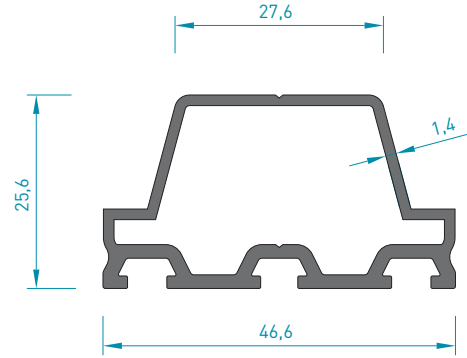
2493 ALT BAĞLANTI PROFİLİ 0.640 kg/mt
