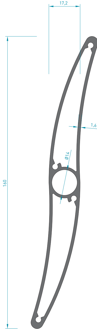
5431 GÜNEŞ KIRICI PROFİLİ 1.700 kg/mt Jx : 134.26 cm 4 Jy : 2.23 cm 4
