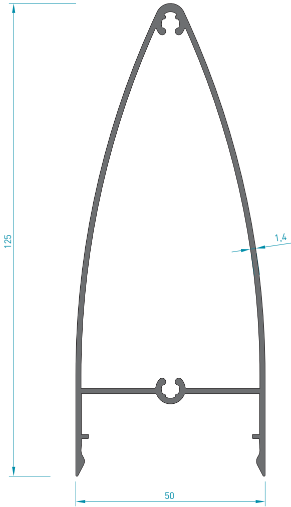
5312 BADEM KAPAK DÜŞEY - YATAY 1.275 kg/mt
