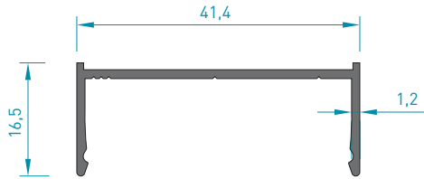
4377 YAN ÇITA (SABİT) 0.245 kg/mt
