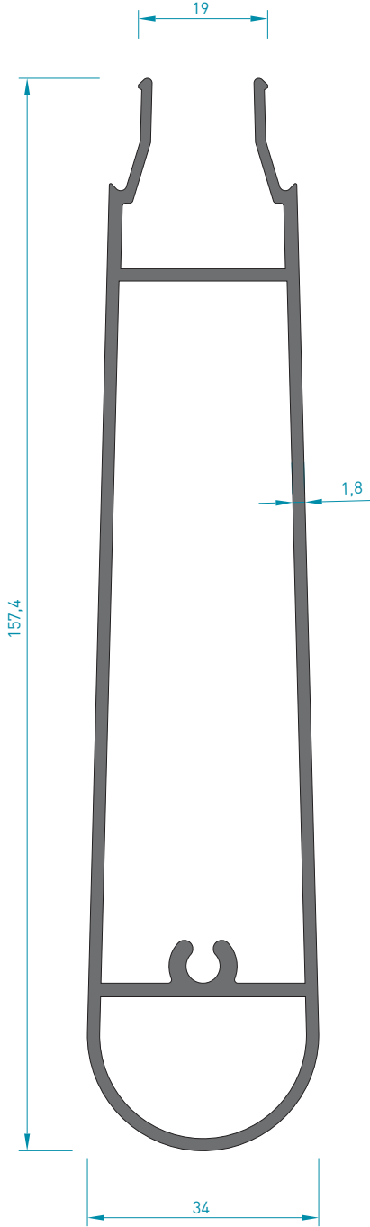
5496 GÜNEŞ KIRICI YAPRAK PROFİL 2.000 kg/mt Jx : 168.76 cm 4 Jy : 11.87 cm 4
