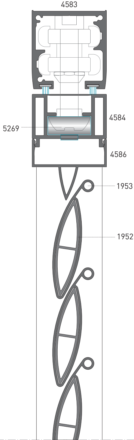
DÜŞEY KESİT (ÜST DETAY)
