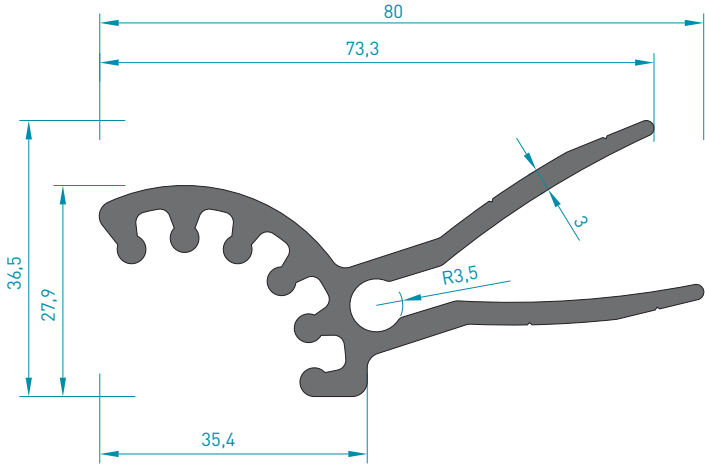
4887 GÜNEŞ KIRICI ÜST BAĞLANTI APARATI 1.445 kg/mt Jx : 21.47 cm 4 Jy : 3.50 cm 4
