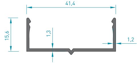
4585 YAN ÇITA (HAREKETLİ) 0.250 kg/mt
