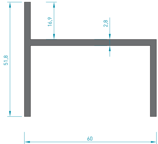
5438 GÜNEŞ KIRICI KASA 1.070 kg/mt Jx : 23.45 cm 4 Jy : 5.51 cm 4
