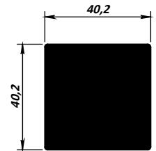
MK-70 - 4,377 kg/m
