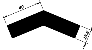
MK-65 - 2,778 kg/m
