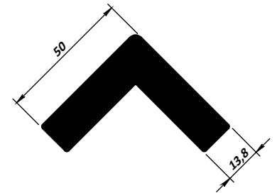
MK-66 - 3,217 kg/m
