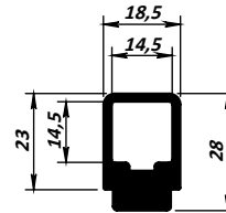
MK-69 - 0,732 kg/m
