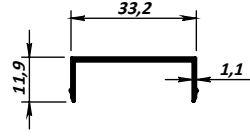
MK-32 - 0,174 kg/m
