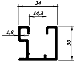
MK-35 - 0,615 kg/m
