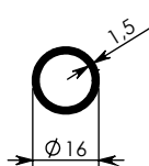
6462 - 0,187 kg/m
