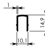
7274 - 0,100 kg/m
