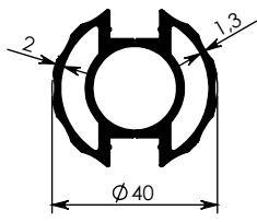
6968 - 0,979 kg/m
