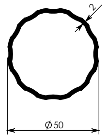
6970 - 0,821 kg/m
