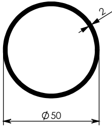
MK-01-A - 0,820 kg/m
