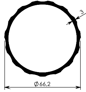
6252 - 1,370 kg/m
