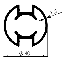
6360 - 0,780 kg/m
