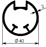
MK-22-D - 0,835 kg/m
