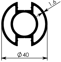
7178 - 0,895 kg/m
