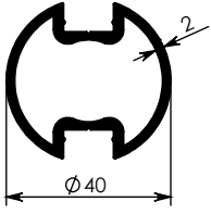
MK-20-D - 0,840 kg/m
