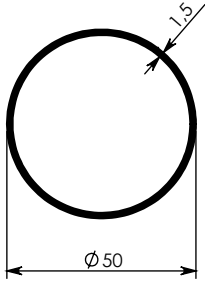
113 - 0,621 kg/m
