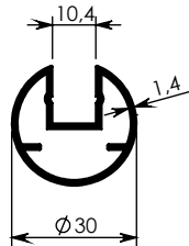
7273 - 0,480 kg/m
