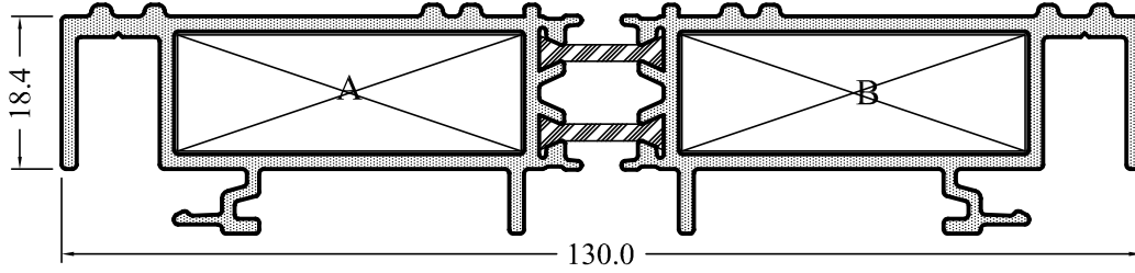
YS1504-18 2,076 kg/m
