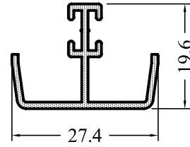
YS1566-12 0,249 kg/m
