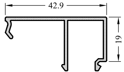
5647-15 0,375 kg/m
