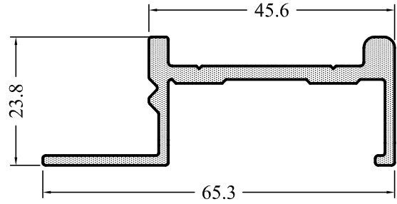
YS1556-18 0,760 kg/m
