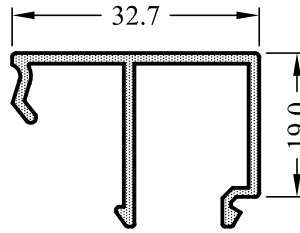
6500-15 0,335 kg/m
