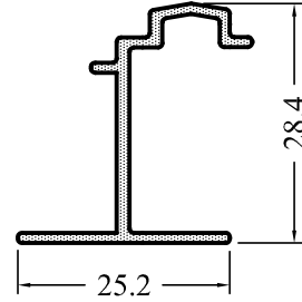
6537-15 0.257 kg/m
