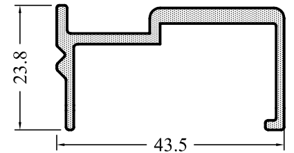
YS1564-15 0,530 kg/m
