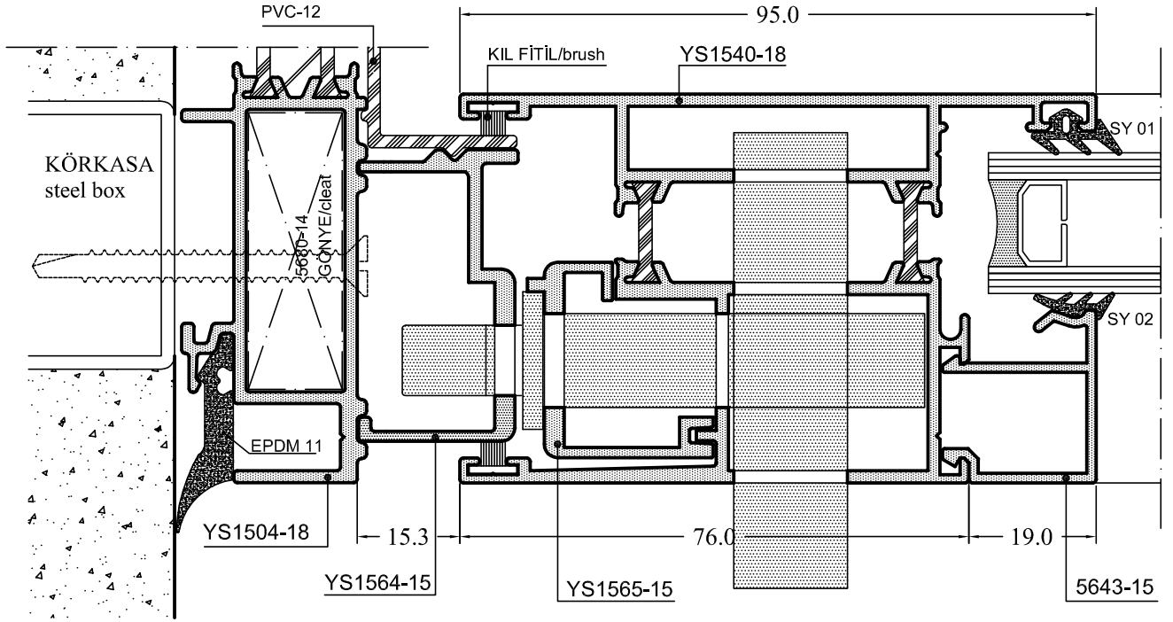
YAN KASA KİLİT YERLEŞTİRME ( 1 )
