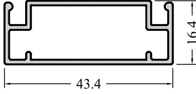
6336-12 0,430 kg/m
