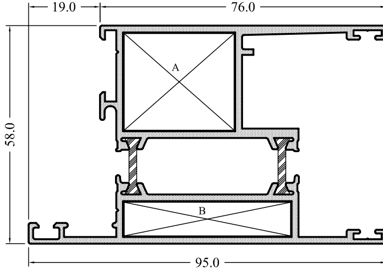
YS1540-18 2,071 kg/m
