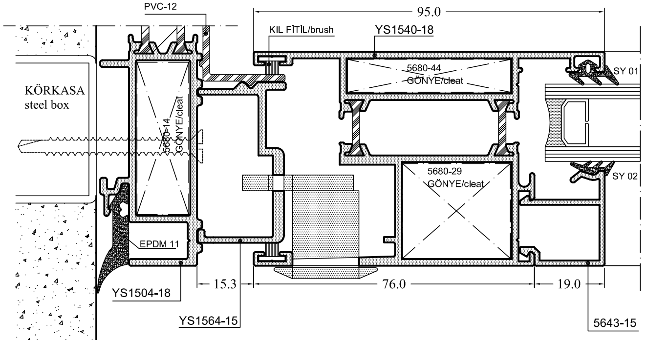
YAN KASA KİLİT YERLEŞTİRME ( 2 )
