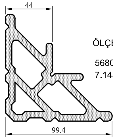
5680-44 7,145 kg/m
