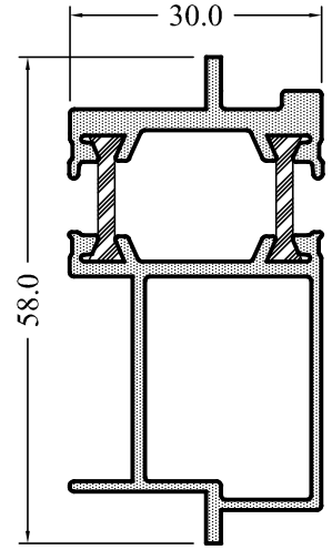
YS1550-12 1,012 kg/m
