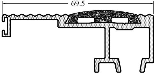
YS1554-20 0,878 kg/m
