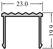
YS1561-10 0,244 kg/m
