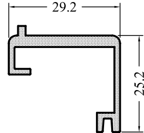
YS1565-15 0,423 kg/m
