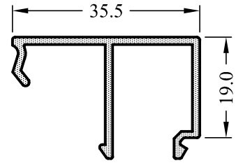
7046-15 0,346 kg/m
