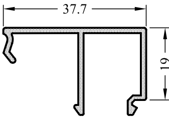
5646-15 0,355 kg/m
