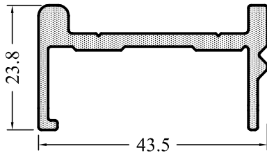
YS1552-18 0,641 kg/m
