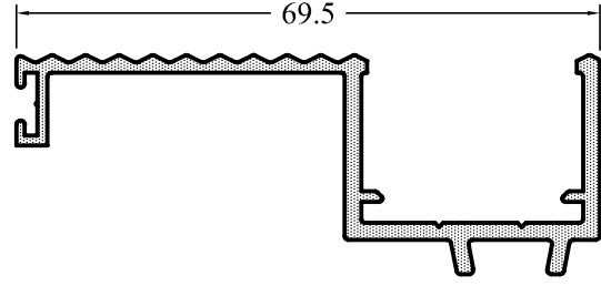
YS1555-20 0,665 kg/m
