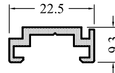
7764 0,209 kg/m
