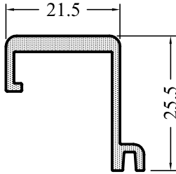
YS1563-15 0,336 kg/m
