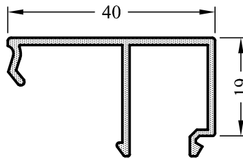
5649-15 0,365 kg/m
