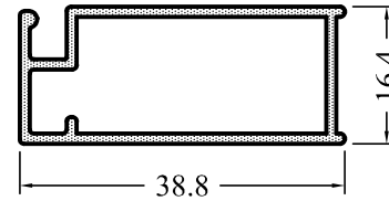
6538-12 0,371 kg/m
