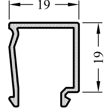
Y55410-15 0,247 kg/m
