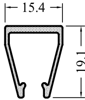
YS1562-18 0,222 kg/m
