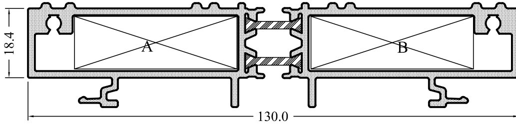
YS1503-18 2,176 kg/m
