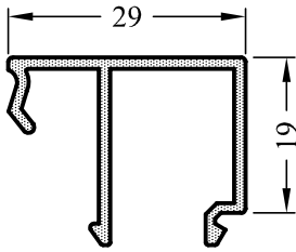
5645-15 0,320 kg/m
