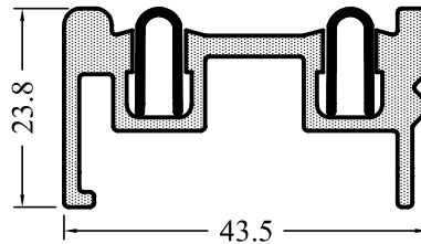
YS1553-18 0,776 kg/m
