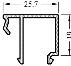
5643-15 0,315 kg/m
