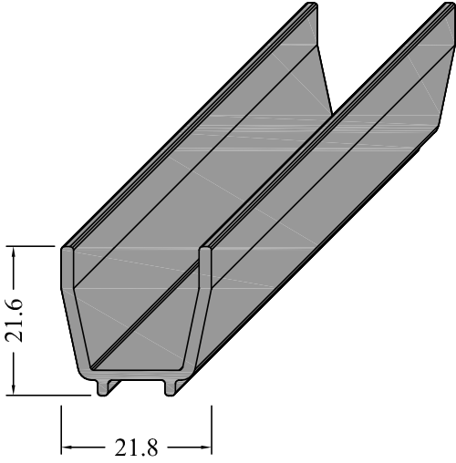
PVC-11 KASA KANAL PLASTİĞİ
