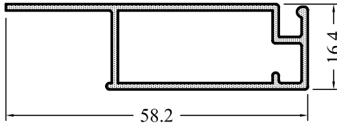
6539-12 0.435 kg/m
