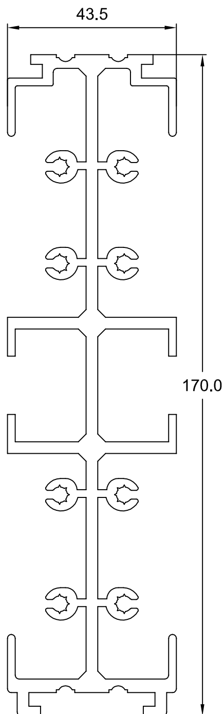
KS-86-00 4.308 Kg/m
