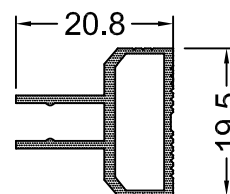
AG 735 0,219 Kg / m
