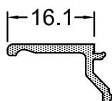
GK58-40 0.113 Kg/m
