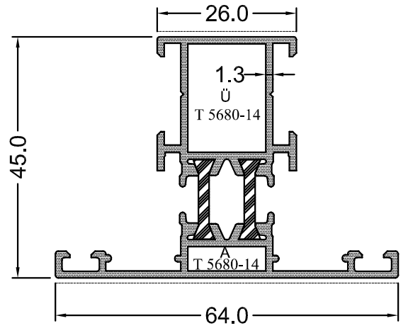
EY4520-13 1.049 Kg/m I_x = 8.06 I_y = 6.08
