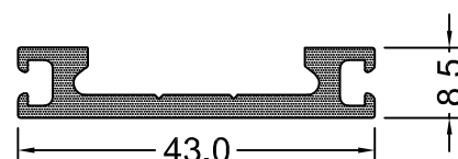
AG-746 0,455 Kg/m
