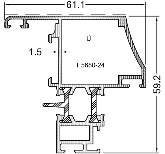
GKS 58-30 1.279 Kg/m
