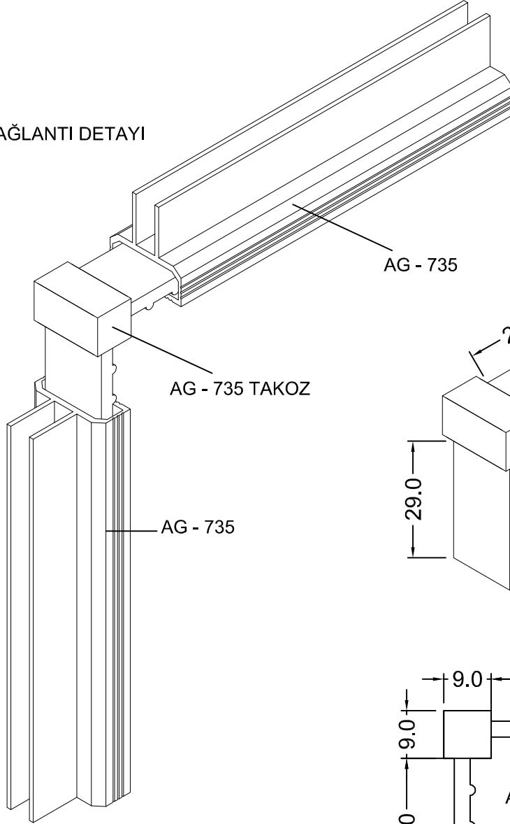
AG - 735 PERPEKTİF DETAYI
