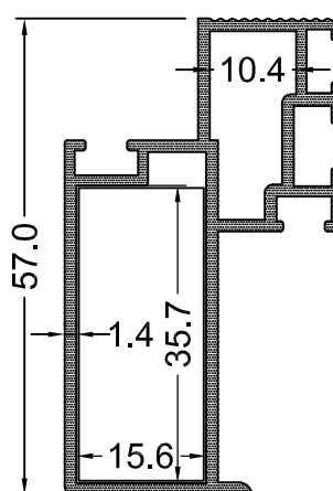
AG 716 - (1695) 0,802 Kg / m
