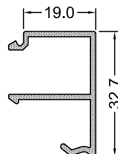
6500-15 0.335 Kg/m
