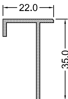
GKS 58-90 0.250 Kg/m
