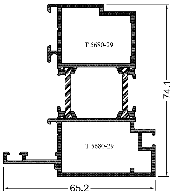
THC.70 1.627 kg /m
