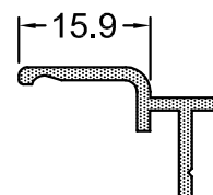
GK58-42 0.170 Kg/m
