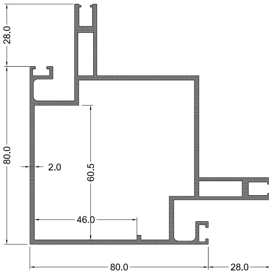
AG 744 2,536 Kg / m
