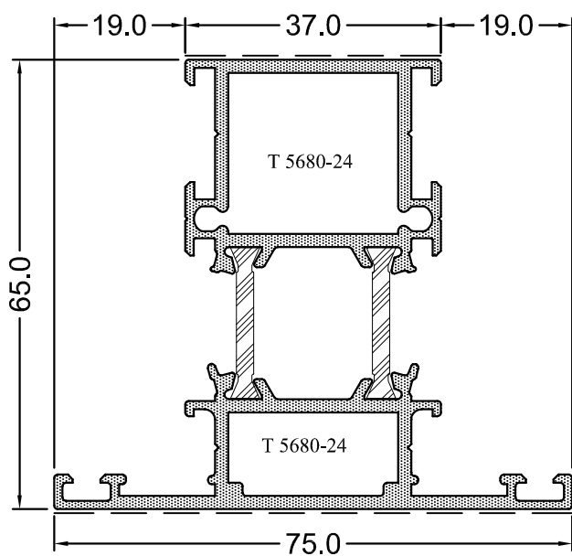
65-RY203-20 1.716 Kg/m
