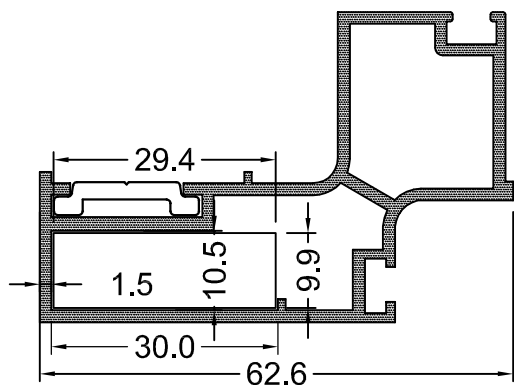
AG 715 0,989 Kg / m
