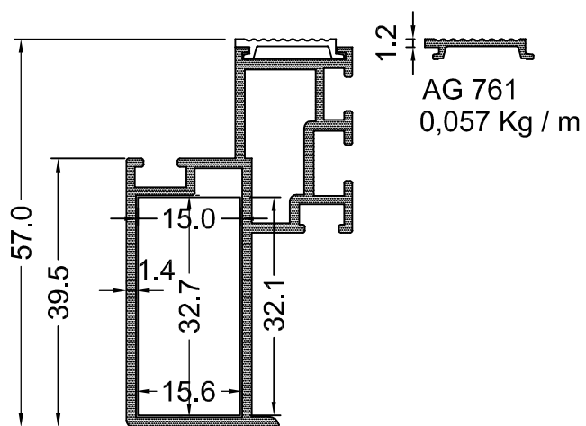
AG 760 0,778 Kg / m
