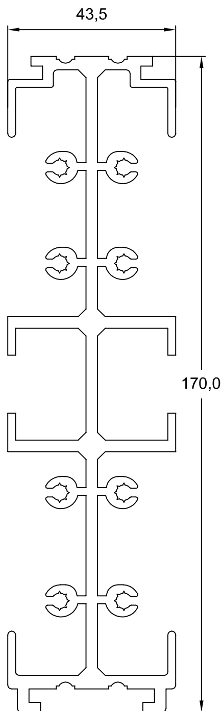
KS-86-00 4.308 Kg/m
