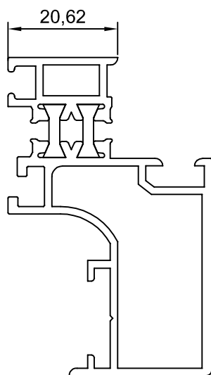
5327-14 1.145 Kg/m
