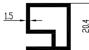
ALS-30 0,353 kg/m
