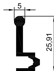
ALS-32 0,271 kg/m
