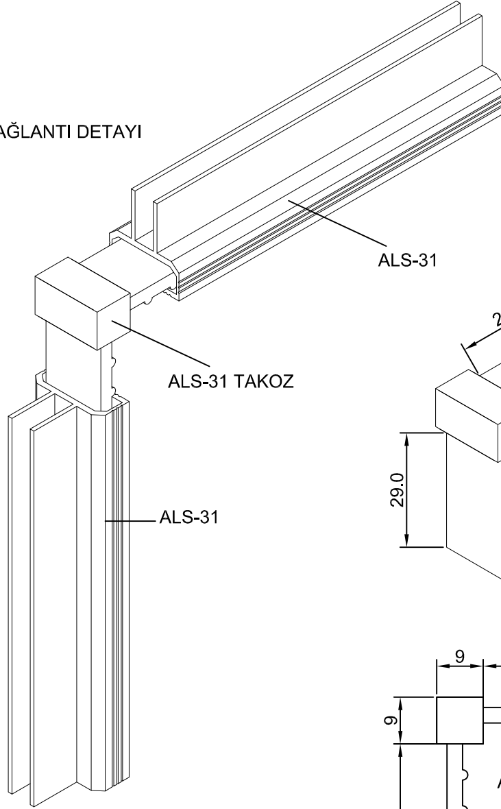
ALS-31 PERPEKTİF DETAYI
