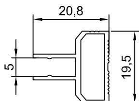
AG 735 0,219 Kg / m
