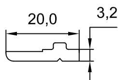
4645-00 0.170 Kg/m
