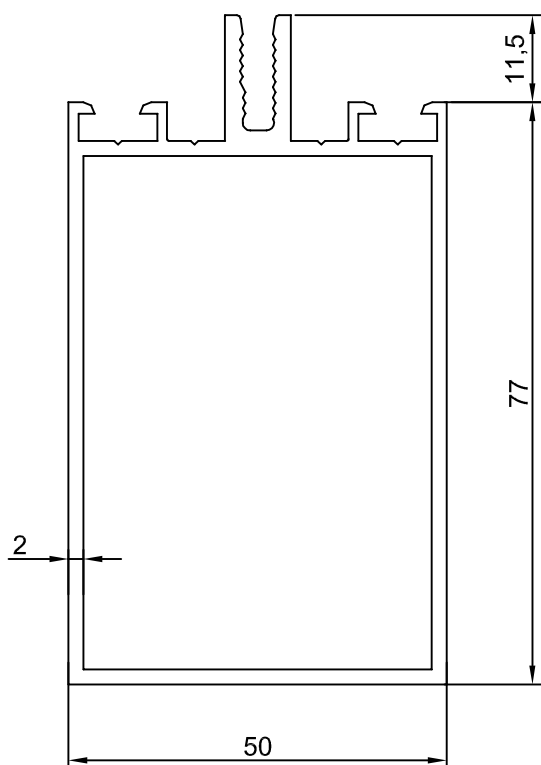
ALS-03 1,594 kg/m Jx:51,77 Jy: 21,32
