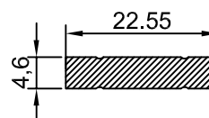
AG 721 0,279 Kg / m
