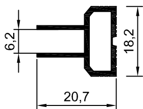
ALS-31 0,220 kg/m
