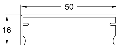
AG 727 6866 - 0,300 Kg / m
