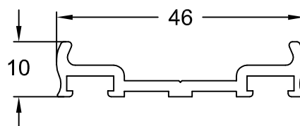
AG 726 6865 - 0,390 Kg / m
