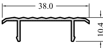
AS-171 0,190 kg/m
