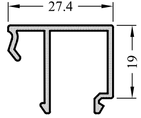
5644-15 0,315 kg/m
