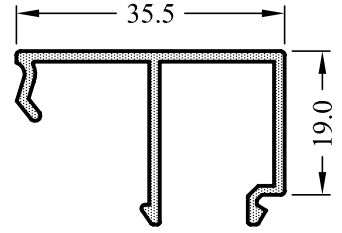
7046-15 0,346 kg/m
