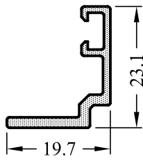
5648-15 0,220 kg/m
