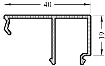
5649-15 0,365 kg/m
