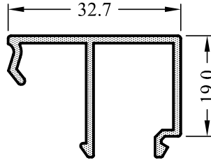
6500-15 0,335 kg/m
