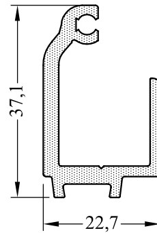
YZÜ5615-00 0,593 kg/m
