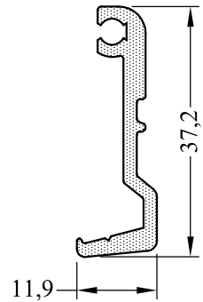
YZÜ5616-00 0,360 kg/m
