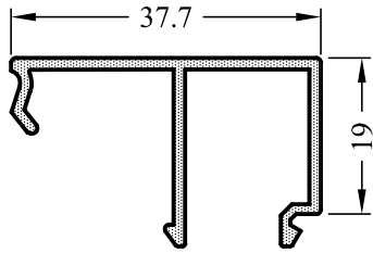
5646-15 0,355 kg/m
