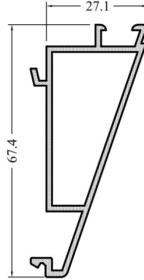
AS-182 0,664 kg/m
