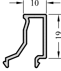
5640-15 0,227 kg/m
