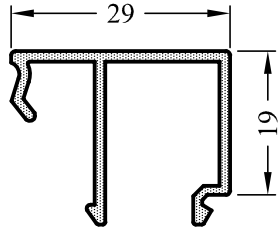
5645-15 0,320 kg/m
