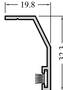
AS-181 0,220 kg/m
