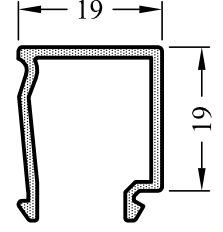
Y55410-15 0,247 kg/m
