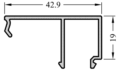
5647-15 0,375 kg/m
