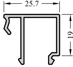
5643-15 0,315 kg/m
