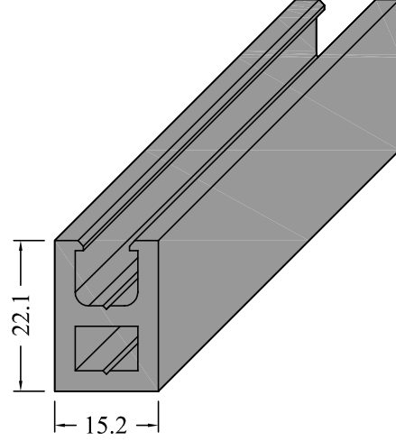
PVC-29 ( Adet ) STOPPER ÜST PLASTİĞİ
