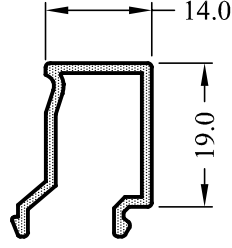
ES4540-13 0,224 kg/m
