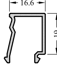
5641-15 0,245 kg/m
