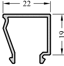
5642-15 0,260 kg/m
