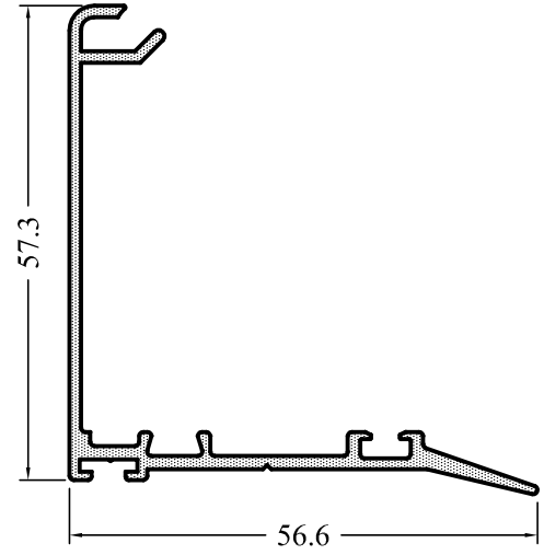
EL47-52 0,580 kg/m
