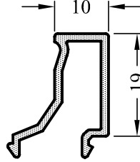
5640-15 0.227 Kg/m
