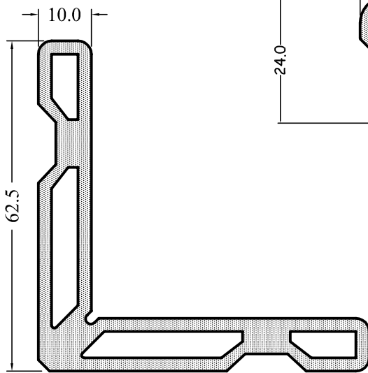
6255-10 1,843 kg/m
