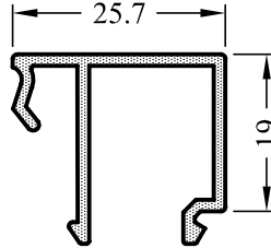
5643-15 0.315 Kg/m
