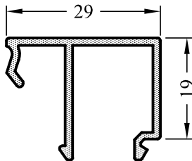
5645-15 0.320 Kg/m
