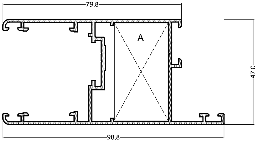
EL47-32 1,273 kg/m
