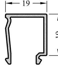
Y55410-15 0.247 Kg/m
