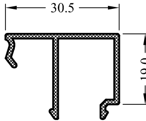
ES4545-13 0.306 Kg/m
