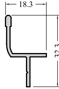
EHS-34 0,205 kg/m
