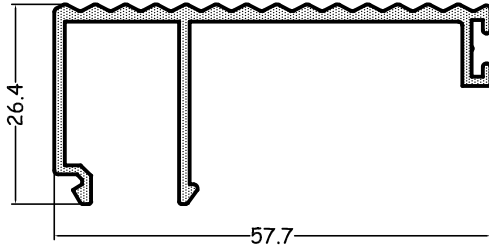
EL47-55-00 0,550 kg/m
