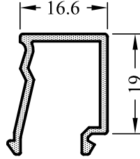
5641-15 0.245 Kg/m
