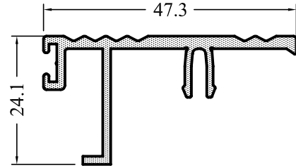
EL47-71 0,485 kg/m
