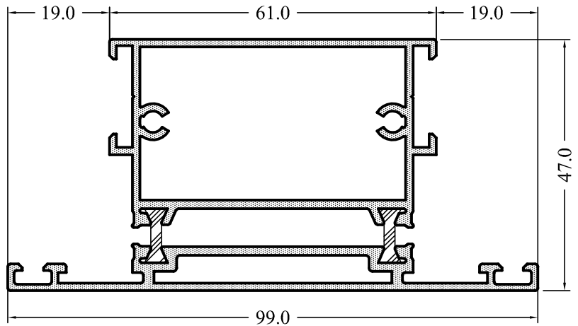
EL47-20 1,753 kg/m
