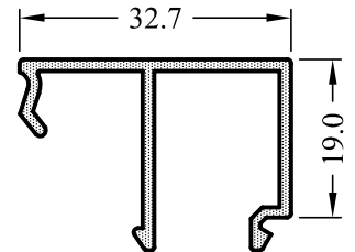
6500-15 0.335 Kg/m
