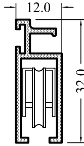
4304-13 0,290 kg/m
