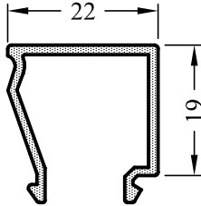
5642-15 0.260 Kg/m
