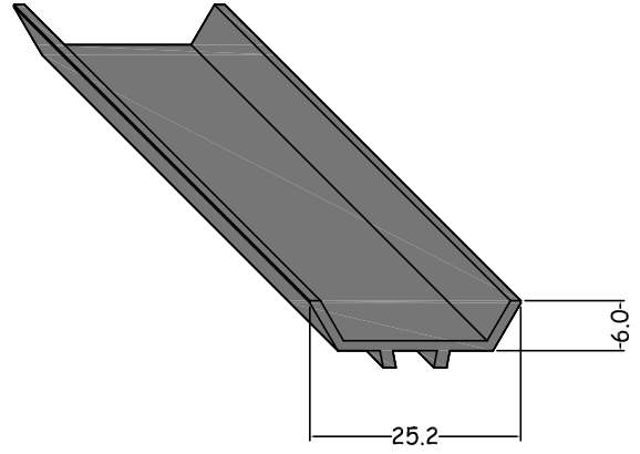
PVC-25 ( Metre ) KASA KANAL PLASTİĞİ ( AS-111 )
