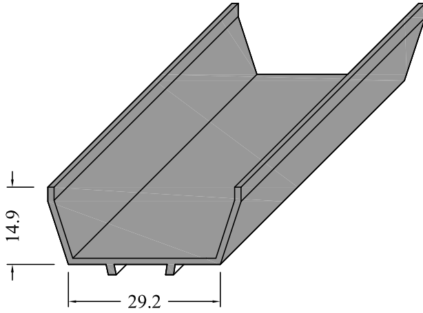
PVC-24 ( Metre ) KASA KANAL PLASTİĞİ ( AS-110 )
