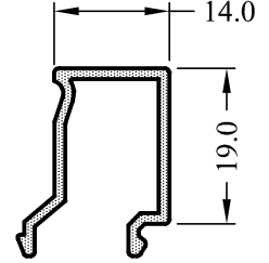
ES4540-13 0.224 Kg/m
