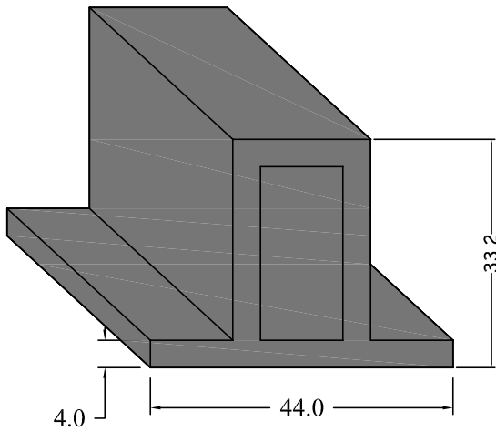
PVC-38 ( Adet ) SABİT KANAT SABİTLEME TAKOZU
