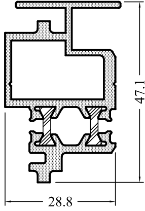
EL47-51 1,085 kg/m
