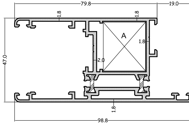
EL47-31-18 1,948 kg/m
