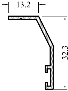
AS-181 0,205 kg/m
