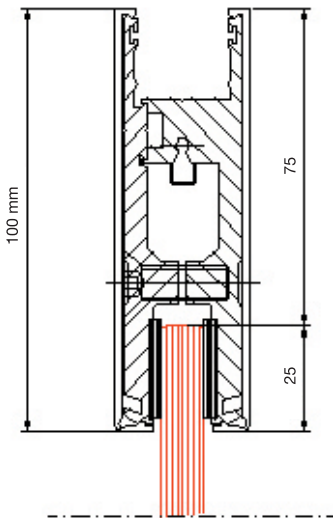
ÜST BAZA İLE TEK KANATLI KAPI
